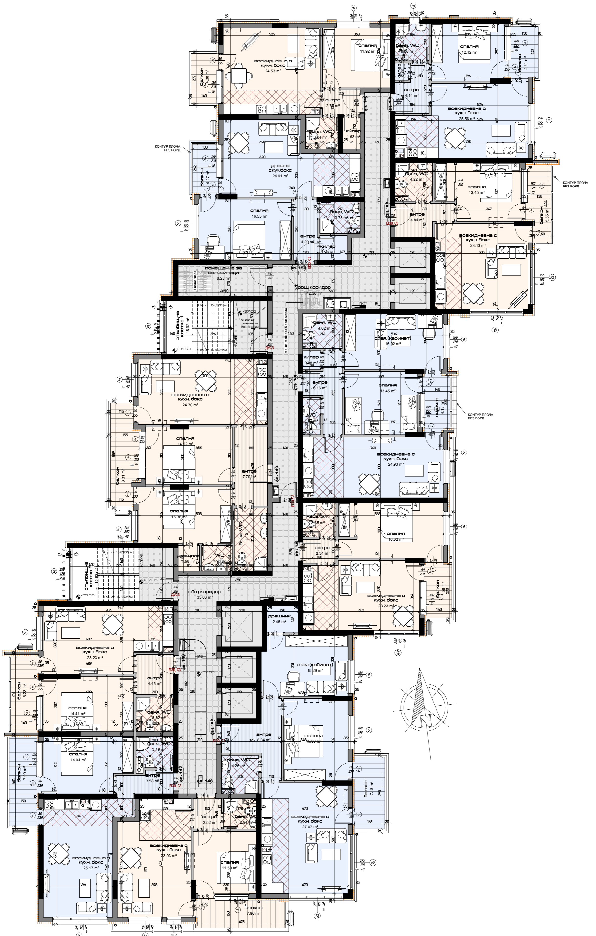
20 РАЗПРЕДЕЛЕНИЕ ЕТАЖ 15 (к.т. +37.05м.)
